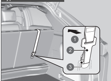
Type met bovenband
